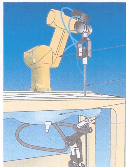
携帯電話端末のSARの測定の様子
